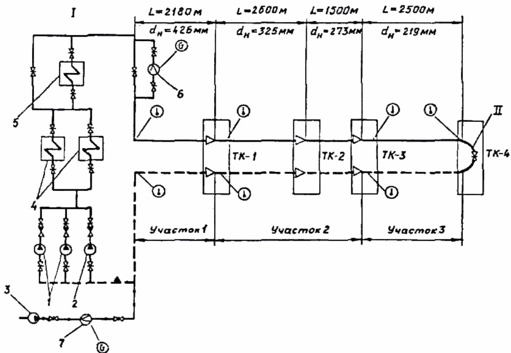
Схема испытываемого циркуляционного кольца
